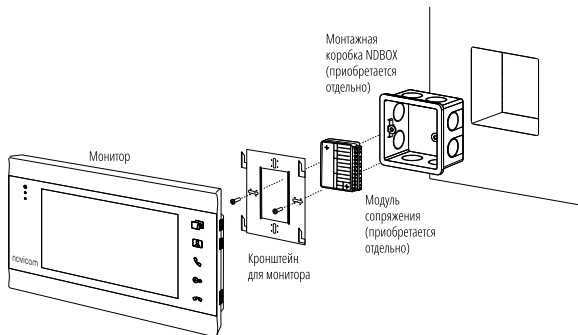
Рис. 6 Монтаж монитора видеодомофона MAGIC
