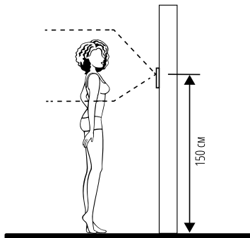
Рис. 5 Рекомендуемая высота установки монитора
