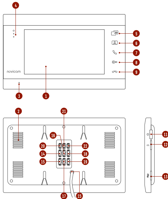
Рис. 3 Описание видеодомофона MAGIC 7 HD
