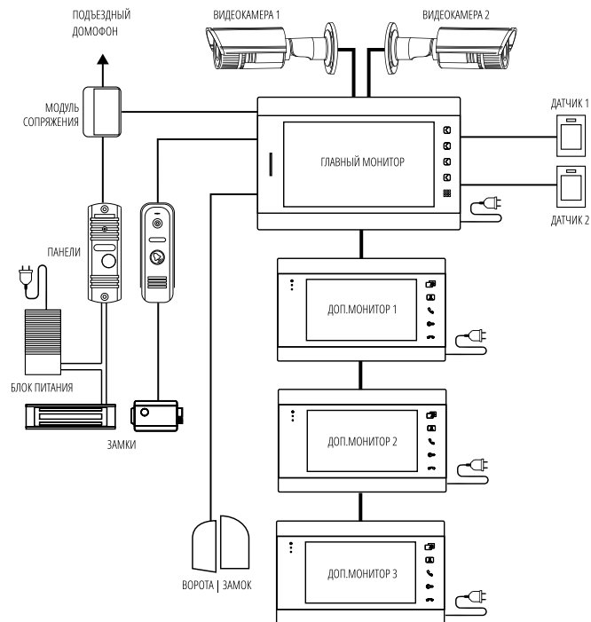
Рис. 10 Функциональная схема системы на базе видеодомофонов MAGIC HD
