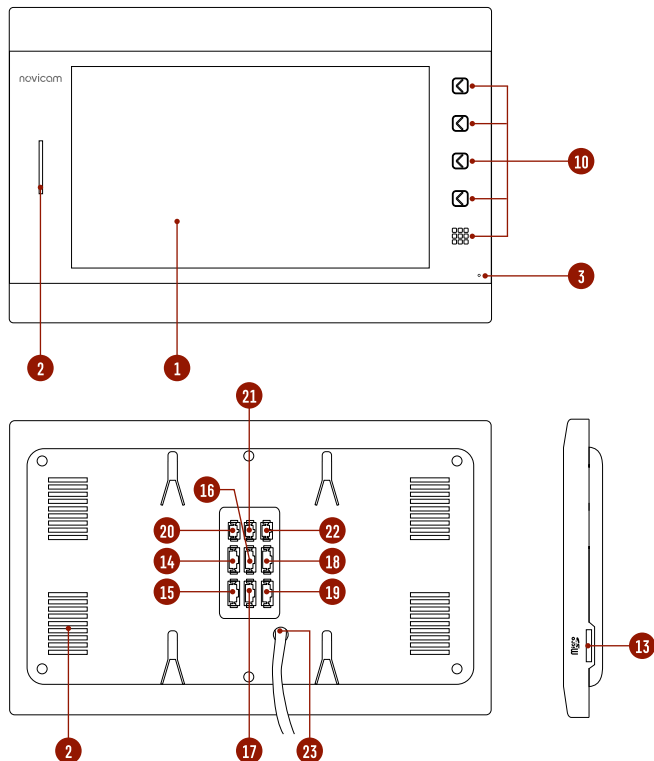
Рис. 4 Описание видеодомофона MAGIC 10 HD
