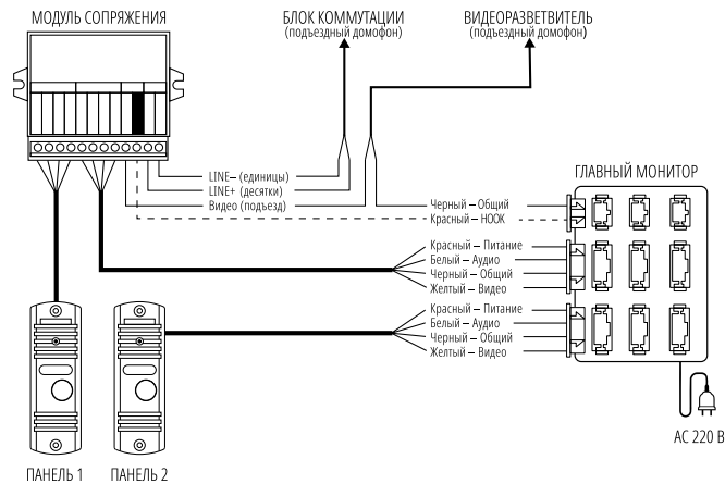
Рис. 12 Схема подключения монитора MAGIC HD к подъездному домофону через модуль сопряжения
