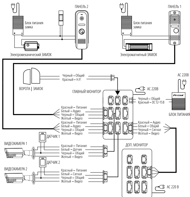
Рис. 11 Схема подключения видеодомофонов MAGIC HD
